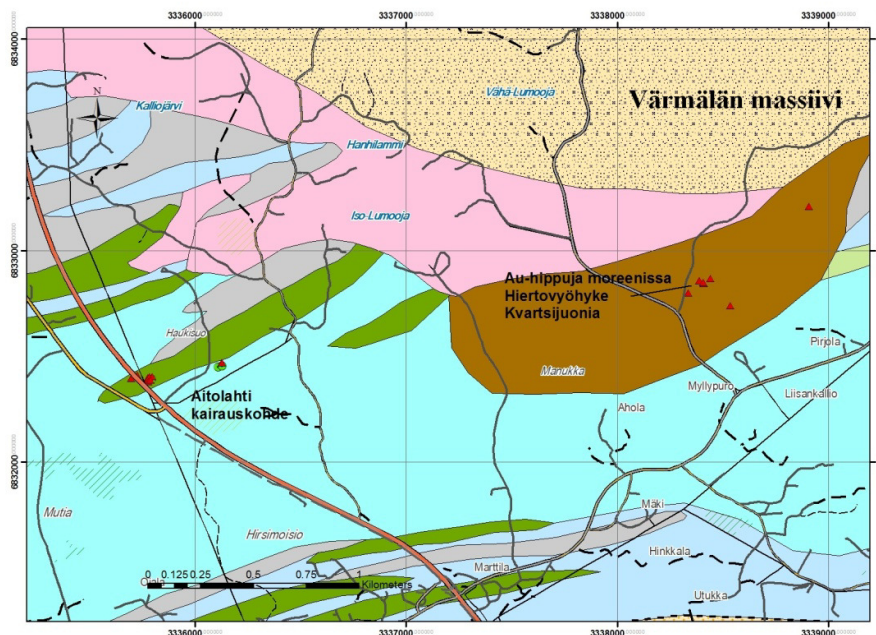
Kuva 7. Aitolahden POKA-kairauskohteen ja itäpuolen gabrointruusiassa oleva Au-kriittisen hieto- ja kvartsijuonivyöhykkeen sijainti kallioperäkartalla (DigiKP-2014).
