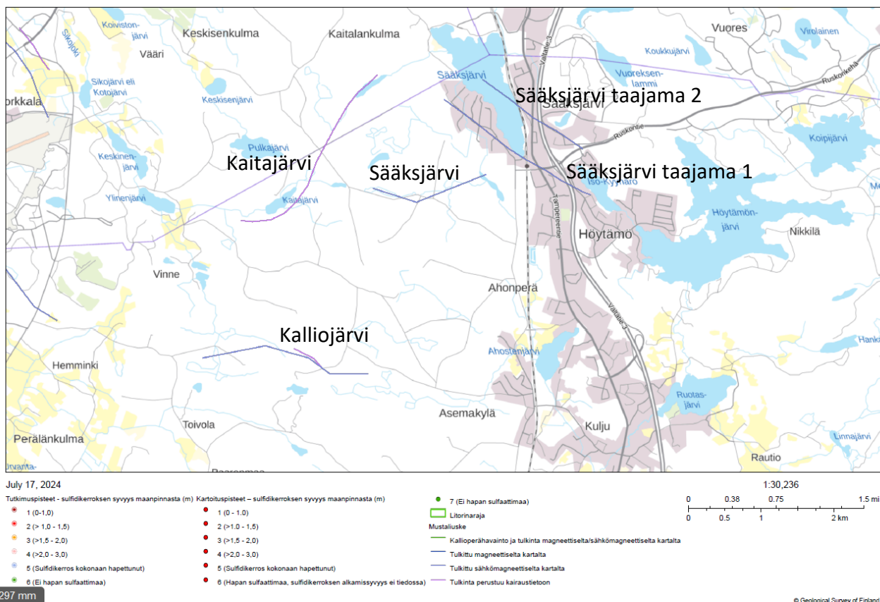
Kuva 4. Tutkimusalueen mustaliuskehavainnot GTK:n happamat sulfaattimaat -palvelusta. Haettu 17.7.2024.
